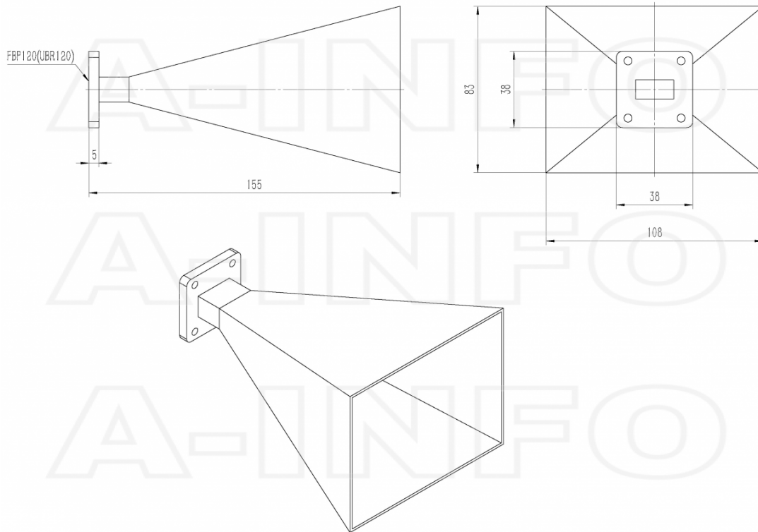
FBP120 Output (P/N: LB-75-20-A)
